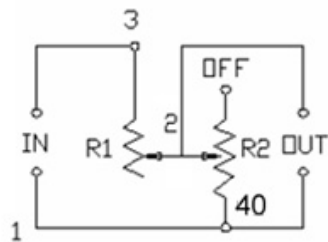
CIRCUIT 電路圖
