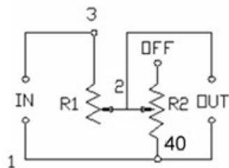
CIRCUIT 電路圖
